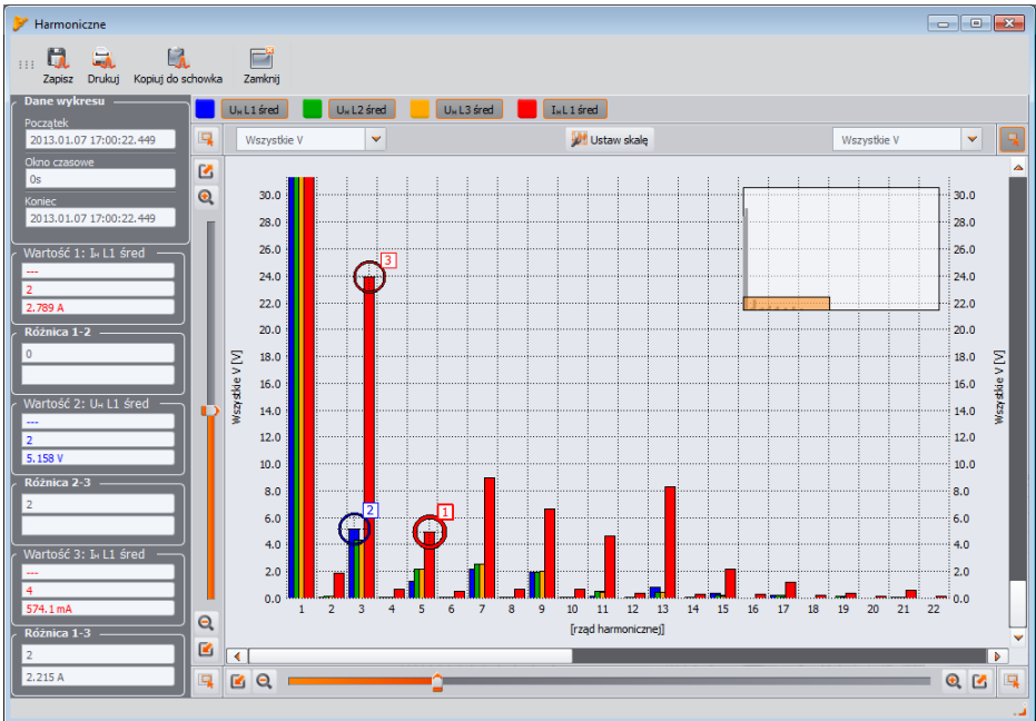
Rys. 62. Wykres harmoniczych.
