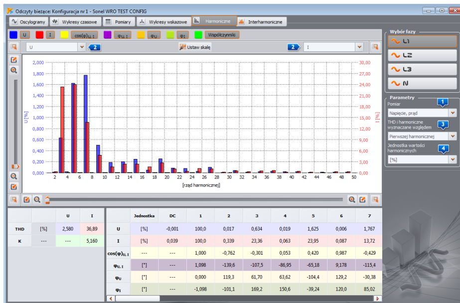
Rys. 51. Bieżące wartości harmoniczych.
