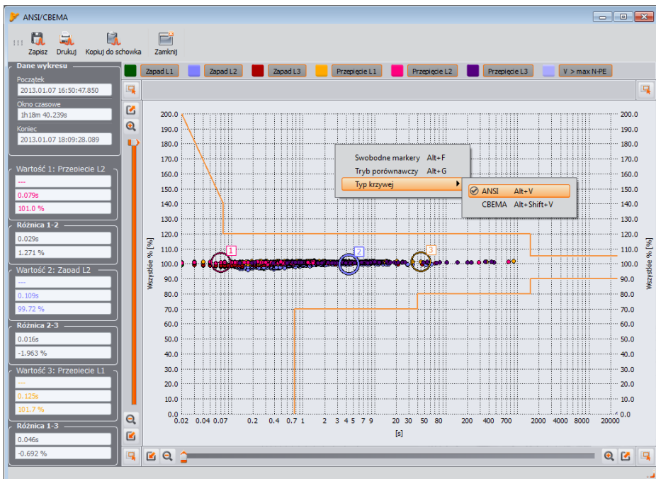
Rys. 72. Wykres ANSI/CBEMA.
