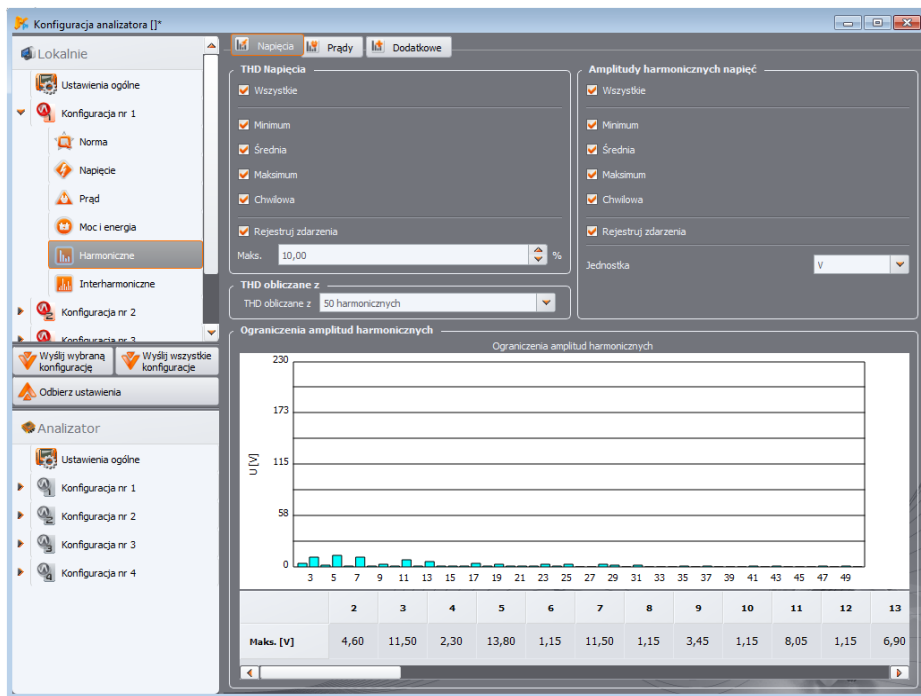
Rys. 29. Ustawienia harmoniczných napięcia.
